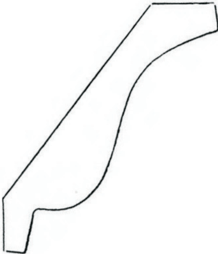
#W-19C 3/4" x 3 1/4"
